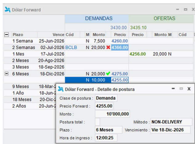
Ilustración 11 Detalle Posturas
